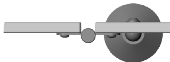
DETAIL A MAßSTAB 1 : 1
