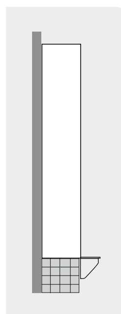
Gemetselde plint met voorgebouwde zitbank
